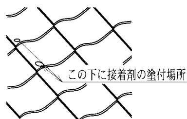
図 -4-18 新しい瓦の取り付け
