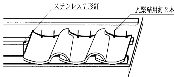
図 -3-12 ステンレス7形釘補強例
