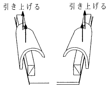
図 -2-24 S形瓦袖瓦の引き上げ例
