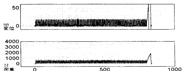
図 - 1-11-B 試験結果
