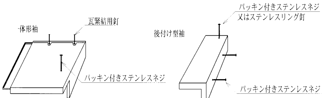
図 -3-18 F形瓦一体型袖瓦の補強例
