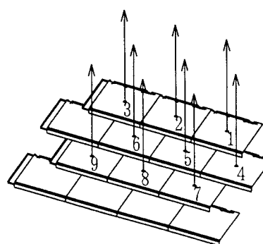
図 - 1-11-A 試験体詳細
