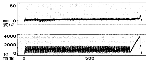
図 - 1-10-B 試験結果
